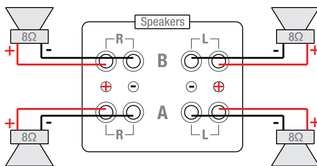
Varianta 1: na každém kanálu prvek s 8\Omega
